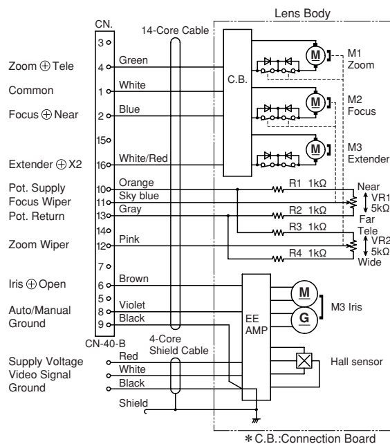
TYPE 2 (DC±12V)
