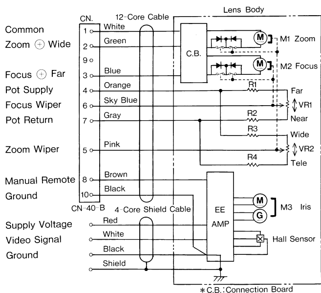
TYPE 3 (DC±6V)
