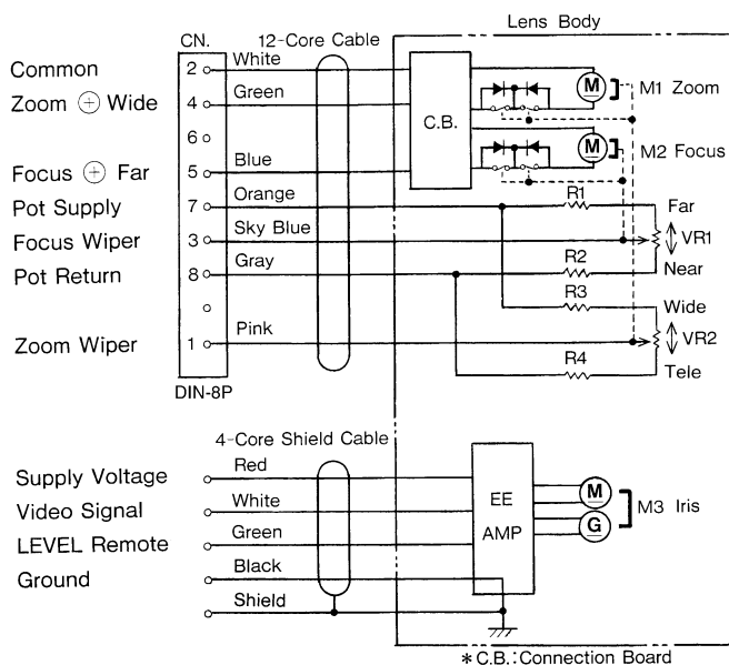
TYPE 3 (DC \pm 6V)
