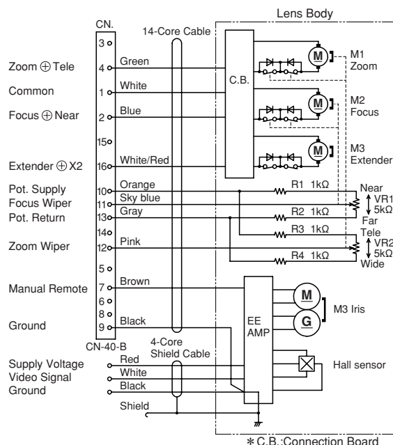
TYPE 2 (DC±12V)
