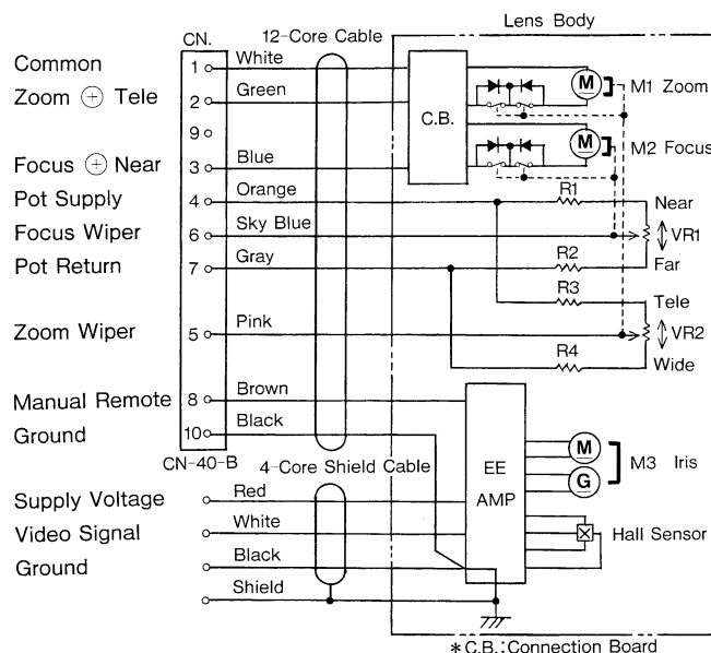
TYPE 2 (DC±12V)
