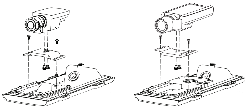
Exemples illustrés : Caméra réseau AXIS M1114 et caisson de protection AXIS T92E05 Caméra réseau AXIS P1343 et caisson d'extérieur AXIS T92E20
