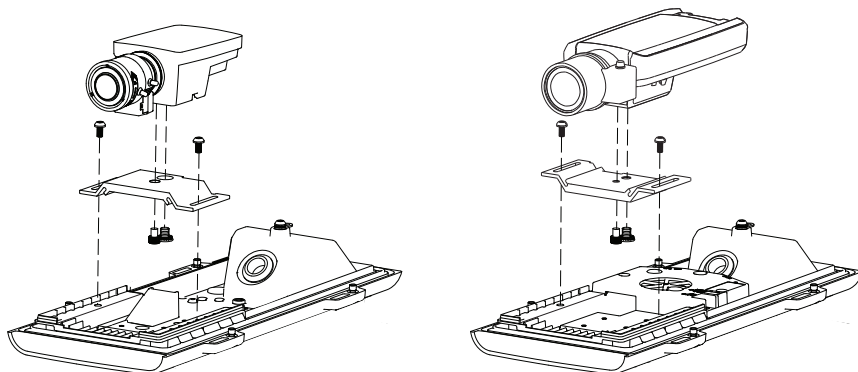
Beispielbilder: AXIS M1114 Netzwerk-Kamera und AXIS T92E05 Schutzgehäuse AXIS P1343 Netzwerk-Kamera und AXIS T92E20 Außengehäuse
