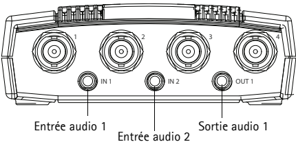
AXIS P7210 – vue arrière
