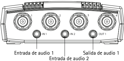
AXIS P7210: vista posterior
