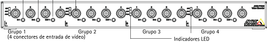
Entradas de audio 1 y 2 Entrada de video AXIS P7210 vista frontal
