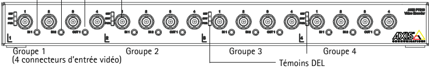
Entrées vidéo 1 et 2 Entrée vidéo AXIS P7210 – vue avant
