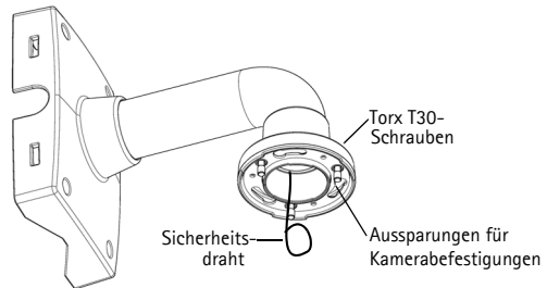
Wandhalterung (Montagebeispiel, Halterung nicht enthalten)
