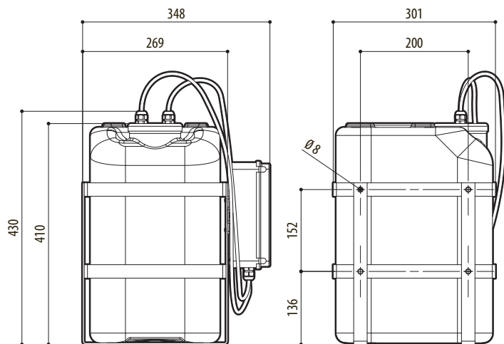
Fig. 49 Réservoir 23l, hauteur de remontée de 5m.
