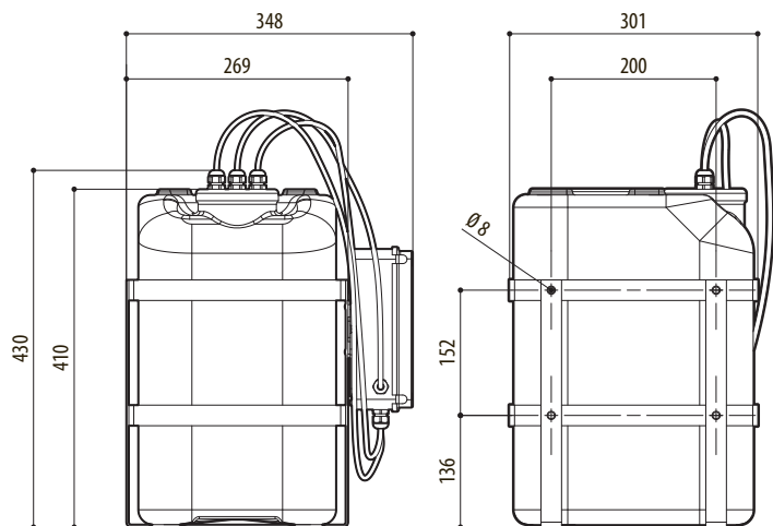
Рис. 50 Канистра 23л, высота напора 11м.
