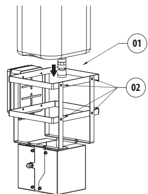
Abb. 5 Wassertank 23l, Förderhöhe 30m.
