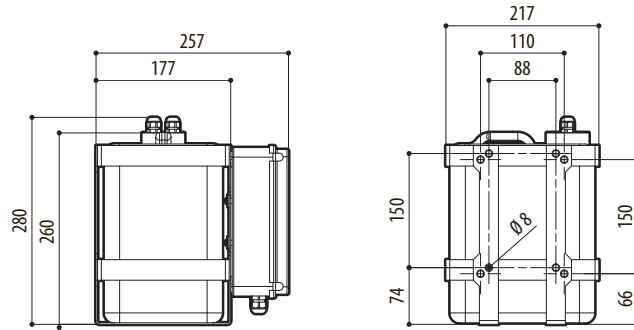
Abb. 48 Wassertank 5l, 5m Förderhöhe.
