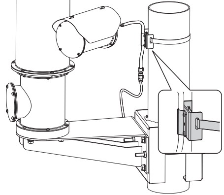
Abb. 46 Montagebeispiel der Scheibenwaschanlage an der Stange.
