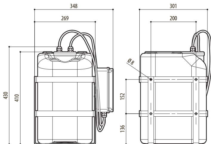
Fig. 49 Tanica 23I, prevalenza 5m.
