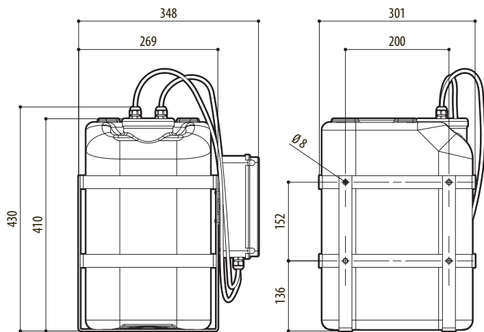
Рис. 49 Канистра 23л, высота напора 5м.
