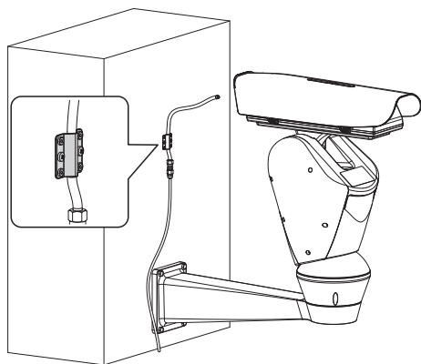
Fig. 45 Esempio di installazione del lavavetro a parete.
