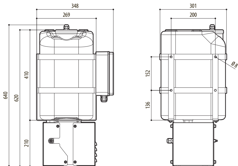
Fig. 51 Tanica 23I, prevalenza 30m.
