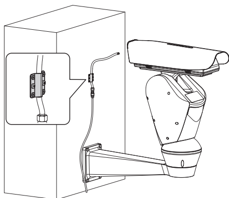
Fig. 45 Exemple d'installation du lave-vitre sur mur.
