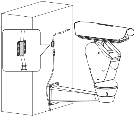
Abb. 45 Montagebeispiel der Scheibenwaschanlage an der Wand.
