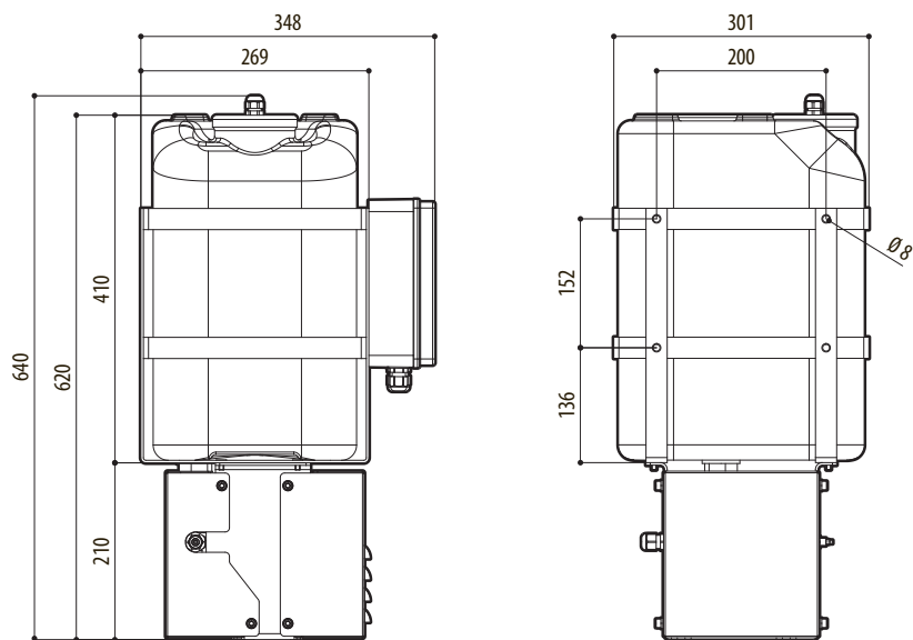
Рис. 51 Канистра 23л, высота напора 30м.
