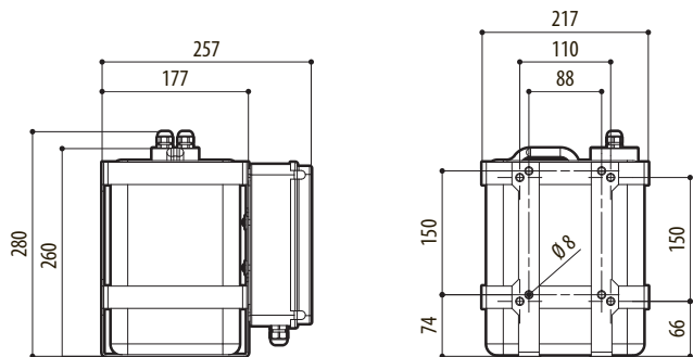
Рис. 48 Канистра 5л, высота напора 5м.
