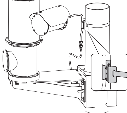
Рис. 46 Пример установки омывателя на опору.
