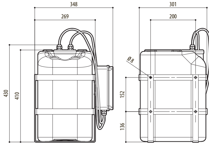
Abb. 49 Wassertank 23l, 5m Förderhöhe.
