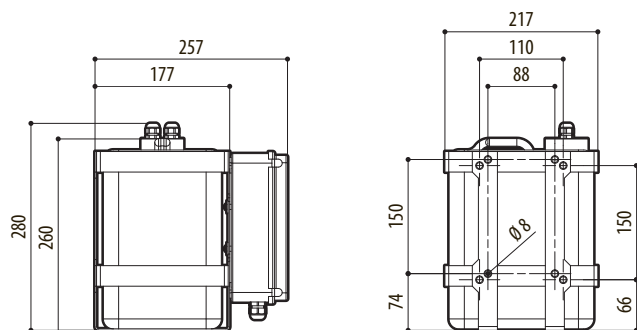
Fig. 48 Tanica 5I, prevalenza 5m.
