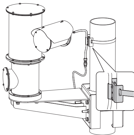
Fig. 46 Esempio di installazione del lavavetro a palo.
