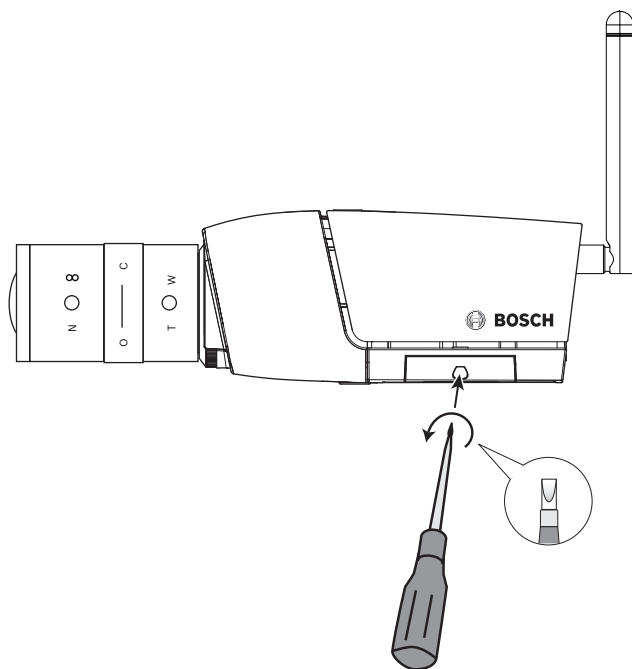
Bild 3.2 SD-Karte
