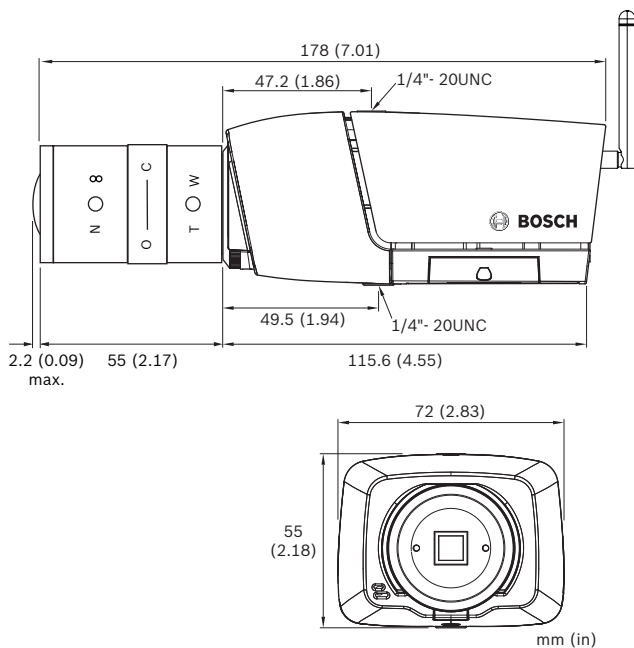
Bild 10.1 Abmessungen
