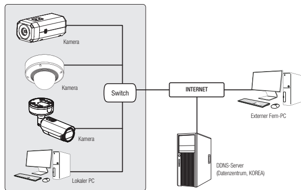
<Lokales Netzwerk>
