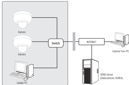
<Lokales Netzwerk>
