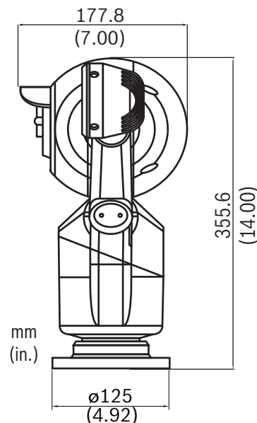
Frontansicht, 90° (aufrecht)
