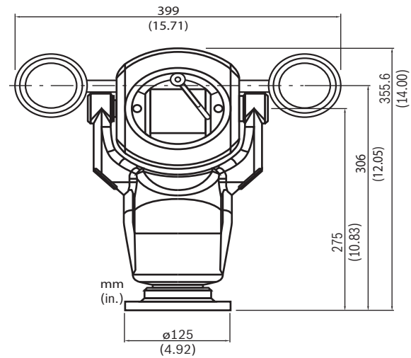
Frontansicht, 90° (aufrecht)
