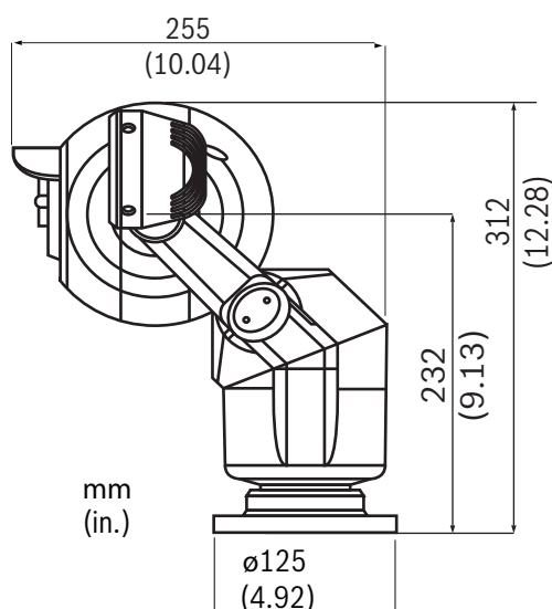
Seitenansicht, 45° (abgewinkelt)
