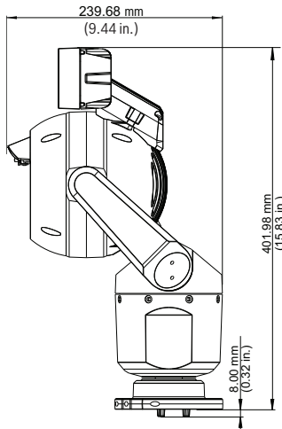
Zijaanzicht, met straler - gekanteld
