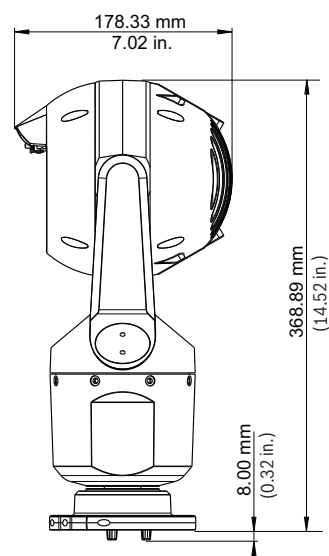
Zijaanzicht - rechtop
