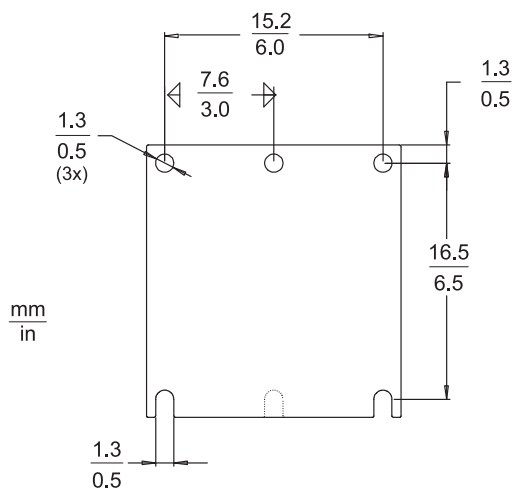
Detaildarstellung B – LTC 9216 und LTC 9222/00 Wandhalterung
