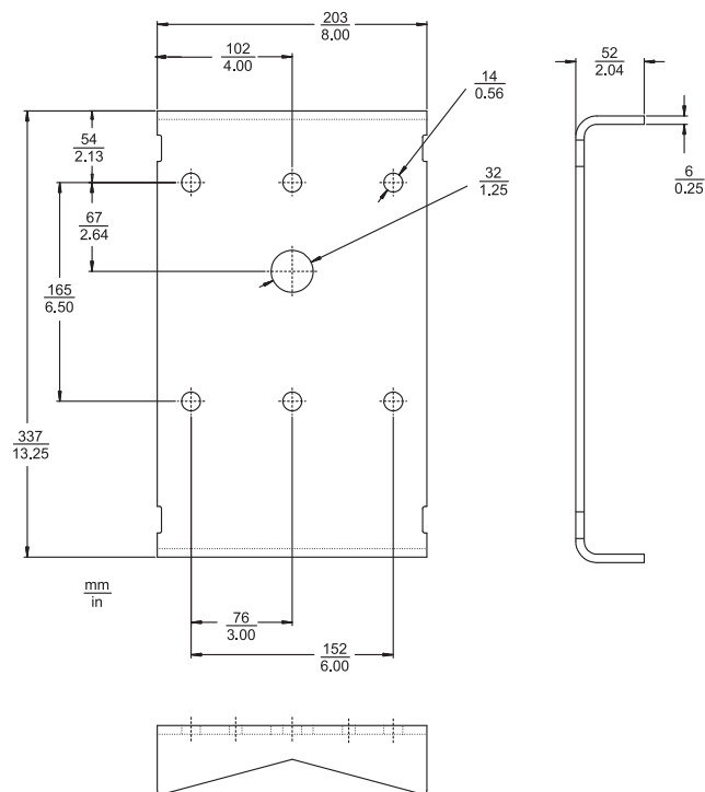
LTC 9225/00 Masthalterung
