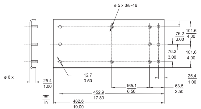
LTC 9228/00 Flanschhalterung
