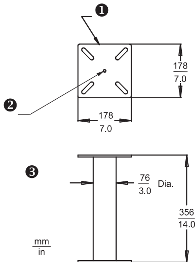
LTC 9214/00 Säulenhalterung, 356 mm
