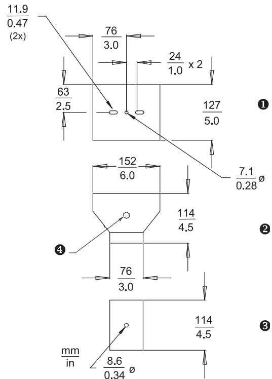
LTC 9227/00 Halterung mit verstellbarem Kopf
