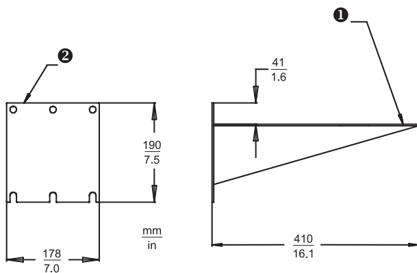
LTC 9216/00 Säulenhalterung, 356 mm
