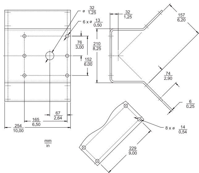
LTC 9226/00 Eckenhalterung
