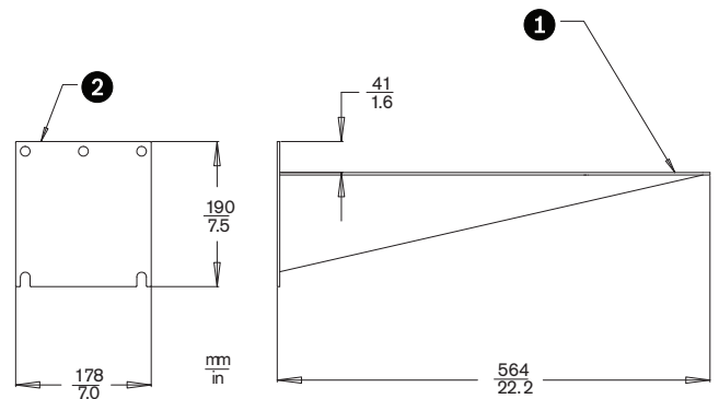
LTC 9222/00 Wandhalterung, 564 mm
