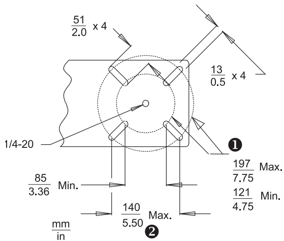
Detaildarstellung A – LTC 9216/00 und LTC 9222/00 Lochkreis-Abbildung
